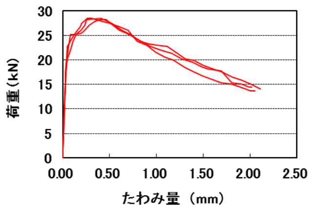
タフネス試験結果 ( \phi 0.7 \times 30 )
